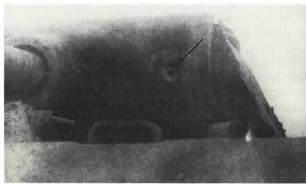
Лобовая броня башни немецкого танка "Пантера" (толщина 100 мм), пробитая 45-мм подкалиберным снарядом (пробитина показана стрелкой)
